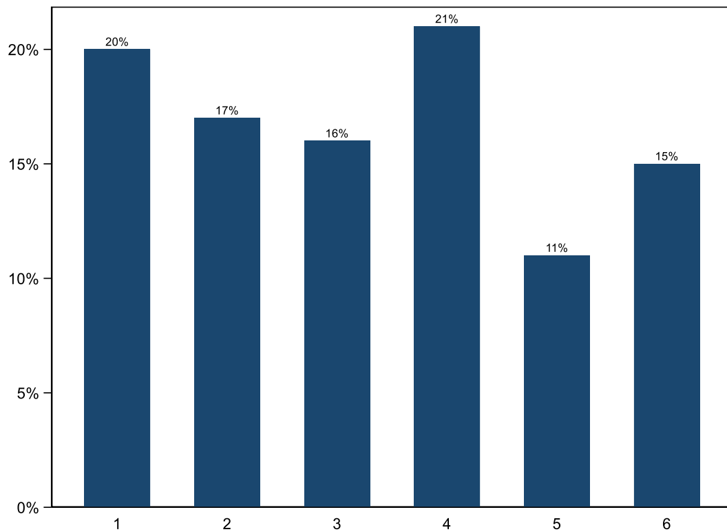
Figura 1. Histograma tirada de un dado con N_{tiradas} = 100 .
