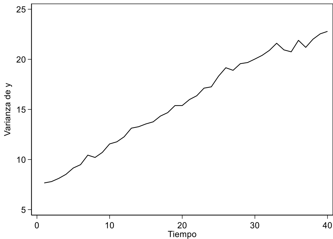
Figura 4. Varianza de ingresos por edad simulada con \rho = 0,9989 .
