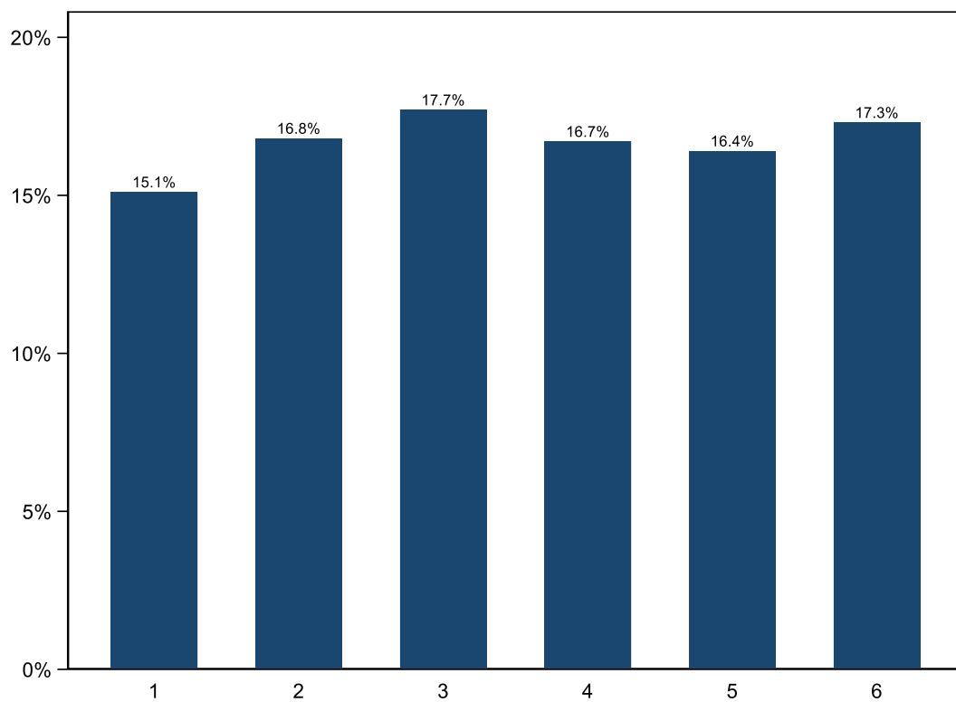
Figura 2. Histograma tirada de un dado con N_{tiradas} = 1.000 .
