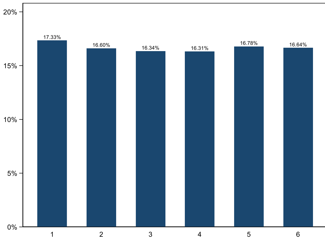
Figura 3. Histograma tirada de un dado con N_{tiradas} = 10.000 .
