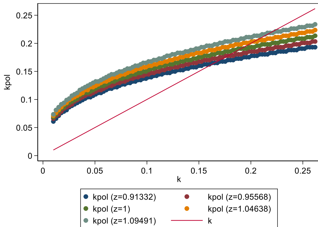
Figura 2. Policy Function de capital para cada valor del shock.
