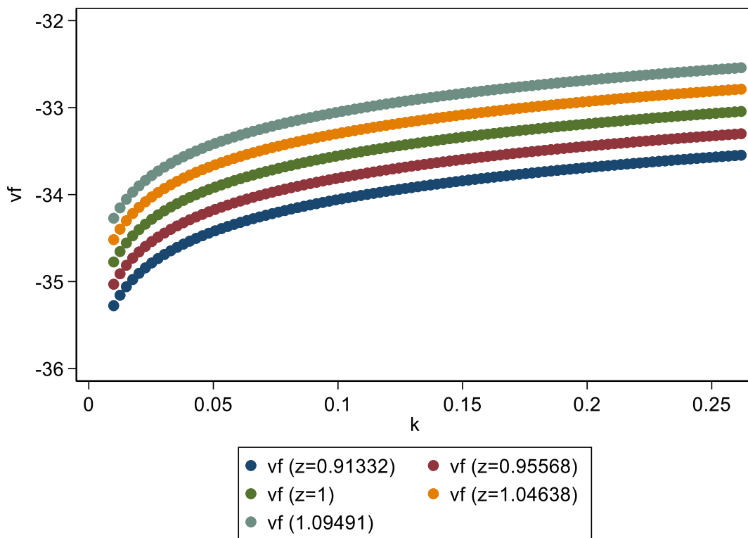
Figura 1. Value Function para cada valor del shock.
